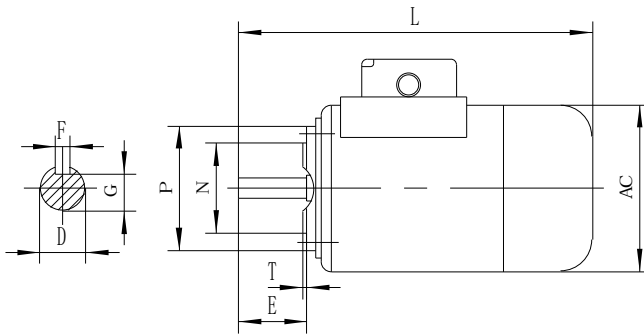
IMB14
