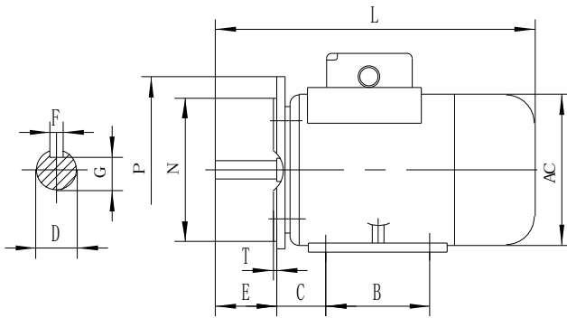
IMB35
