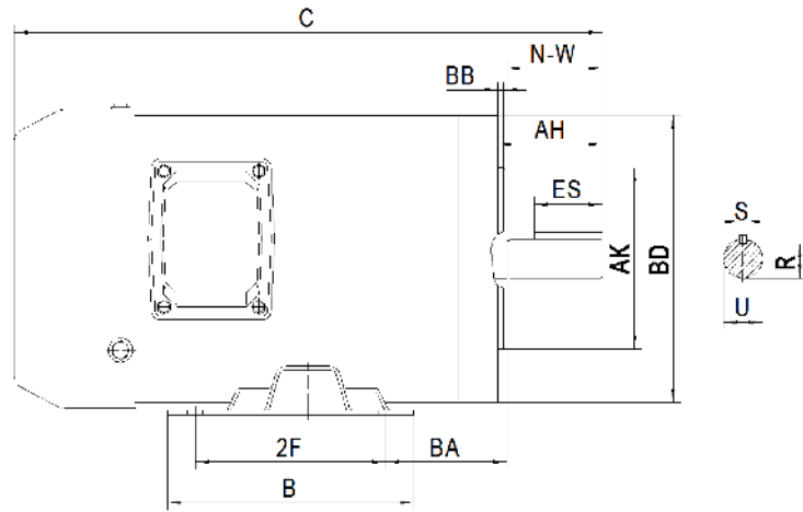
Frame 56-140T
